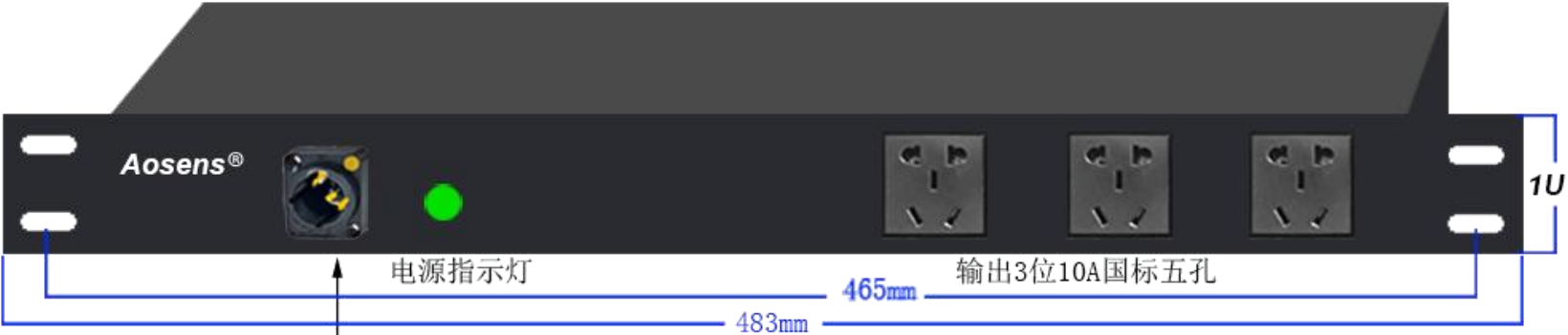
Aosens® 奥盛定制 PDU 示意图
